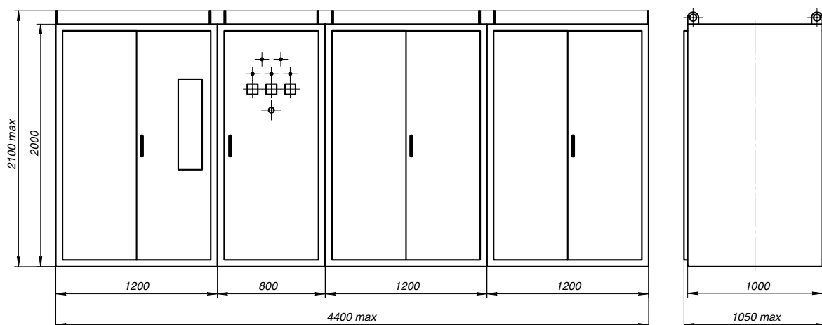
Рисунок 30. Общий вид, габаритные размеры (мм) и масса установки типа УКВ-10,5-4800-2400 УЗ
