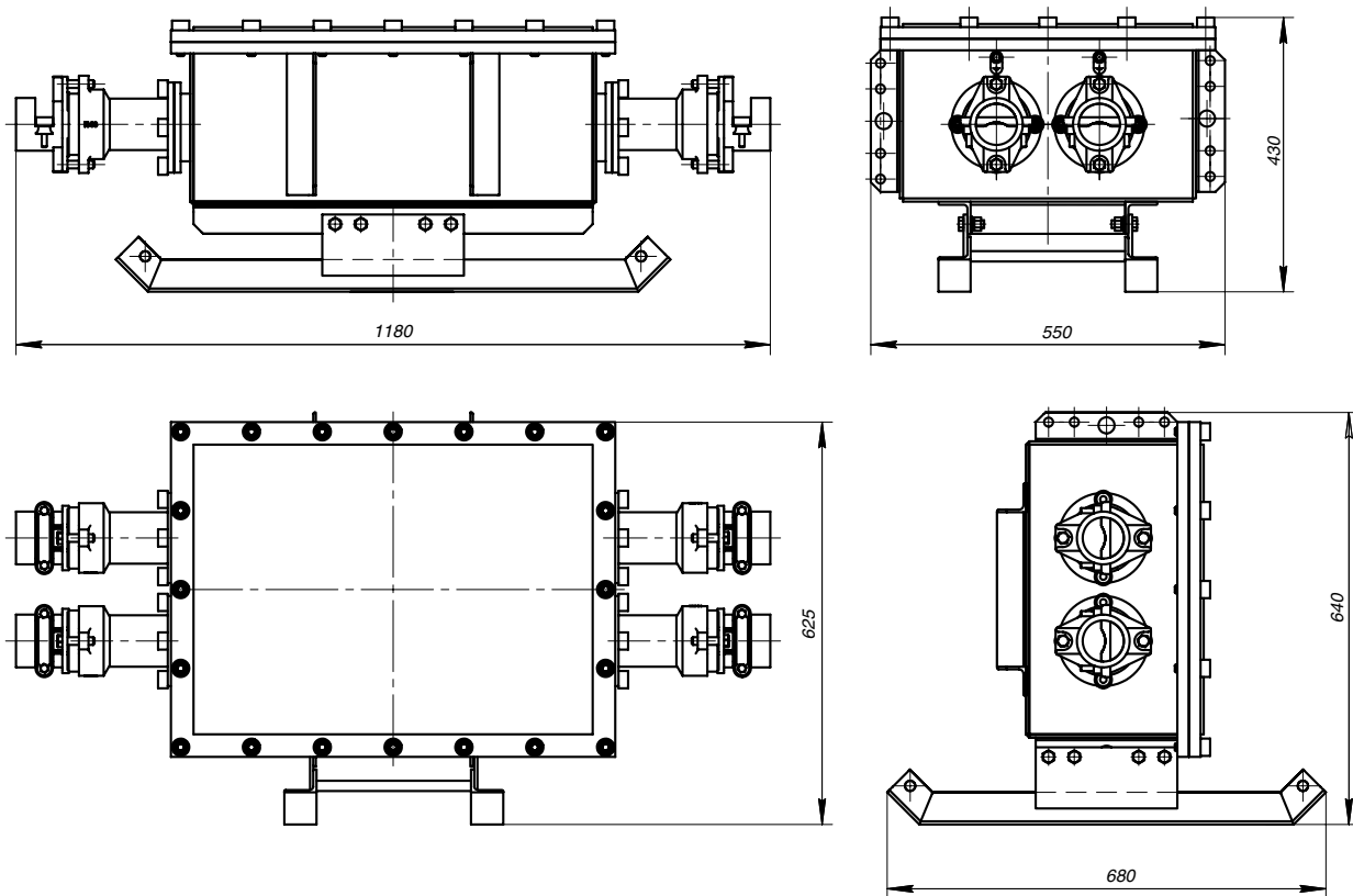
Рисунок 29. Габаритные, установочные размеры (мм) и масса устройства УСВВ
